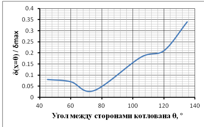
Рис. 8. Фактор №1 в зависимости от угла между сторонами котлована
