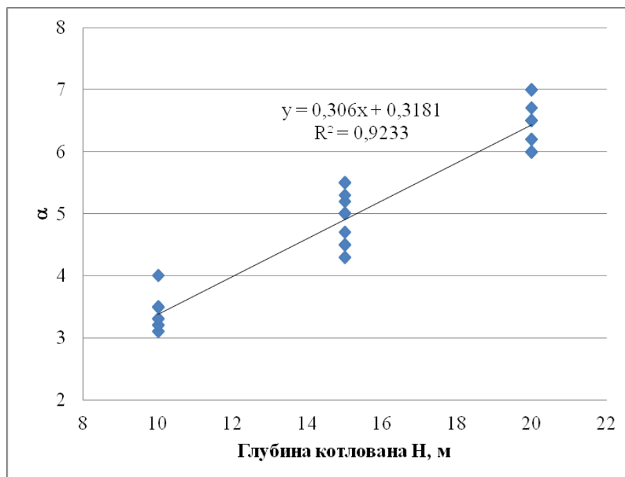
Рис. 2. График зависимости коэффициента \alpha от глубины котлована H
