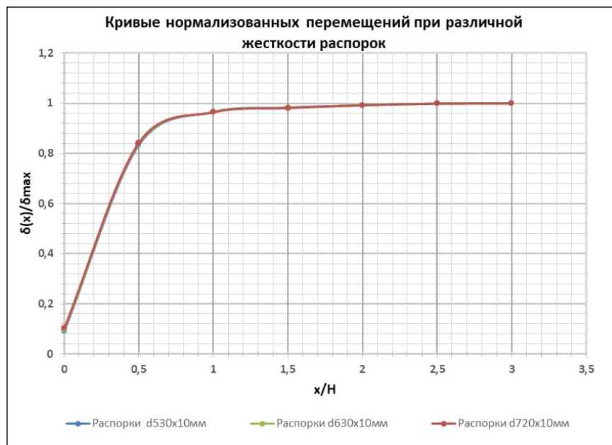
Рис. 12. Кривые нормализованных перемещений при различной жесткости распорок
