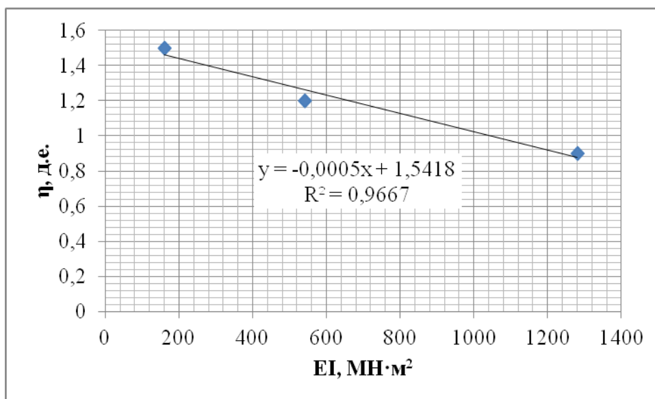
Рис. 14. Зависимость параметра \eta от изгибной жесткости ограждения
